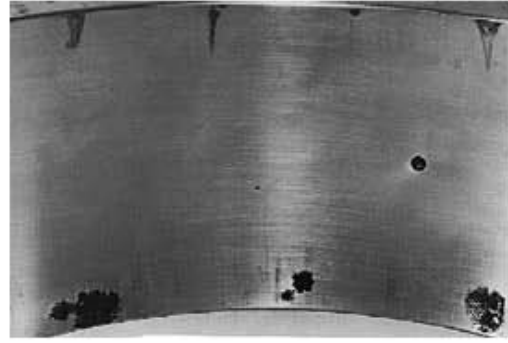
Depoda korozyona uğrama. Aşınma, nemin yoğunlaştığı makara altlarında meydana gelmiş.
